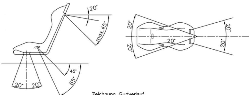
Zeichnung Gurtverlauf
